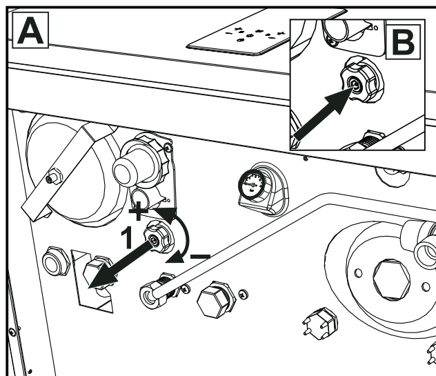
fig. 26- Llave de llenado
