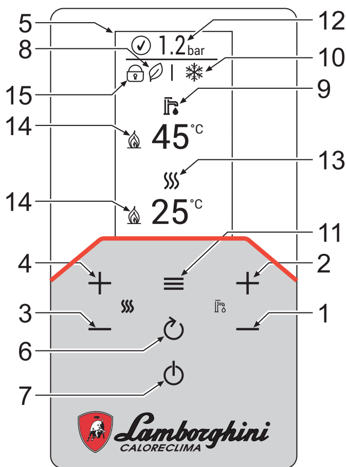
fig. 1- Panoul de control
