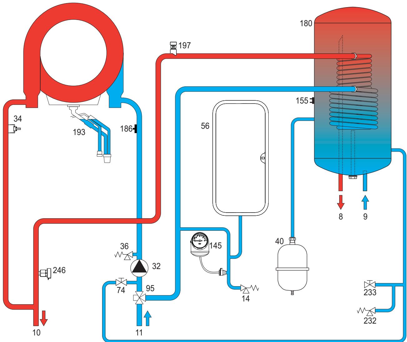
fig. 61- Circuito hidráulico
