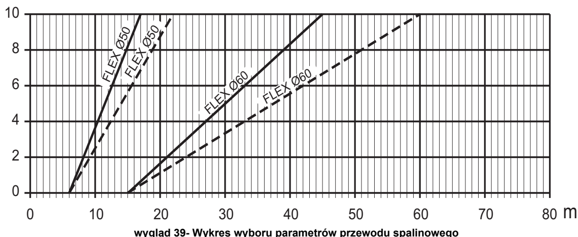
wygląd 39- Wykres wyboru parametrów przewodu spalinowego
