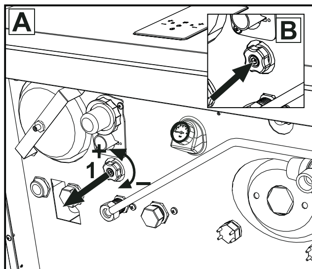
εικ. 26- Διακόπτης πλήρωσης
