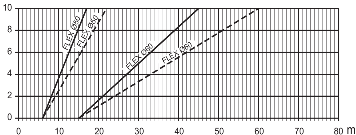
fig. 39- Grafic pentru alegerea parametrului pentru horn
