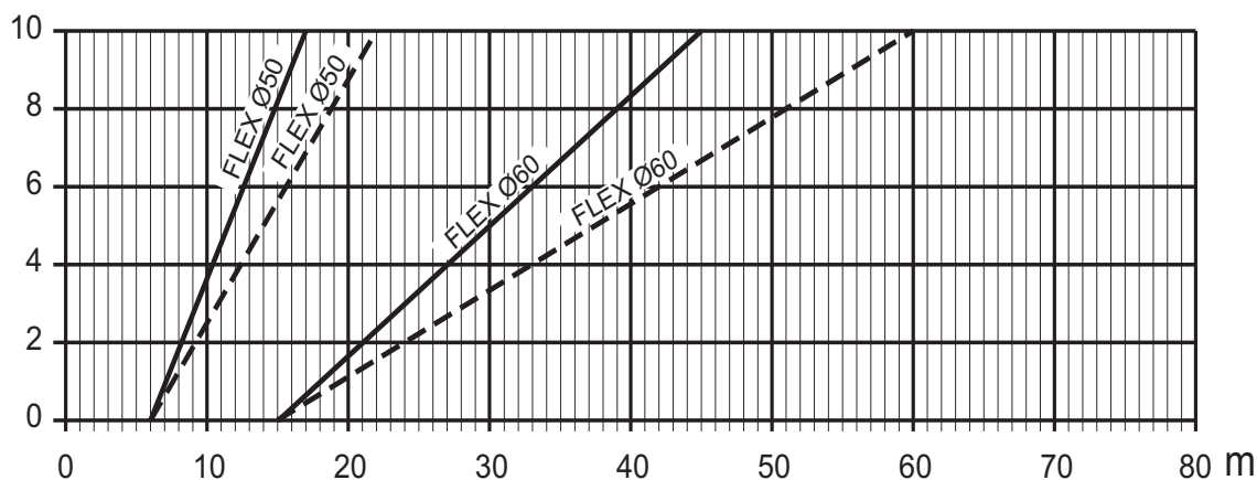
fig. 39 - Grafico per scelta parametro camino
