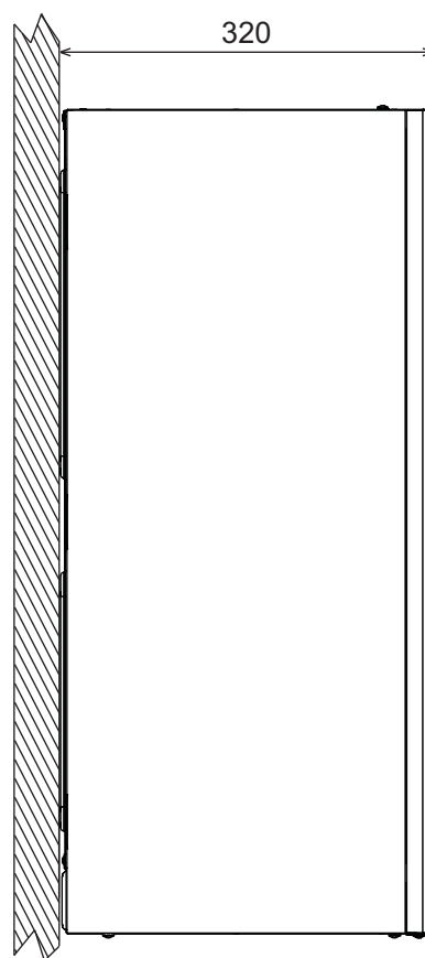
wygląd 57- Widok z boku
