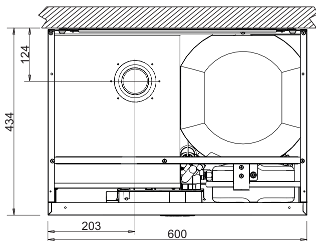
wygląd 58- Widok z góry
