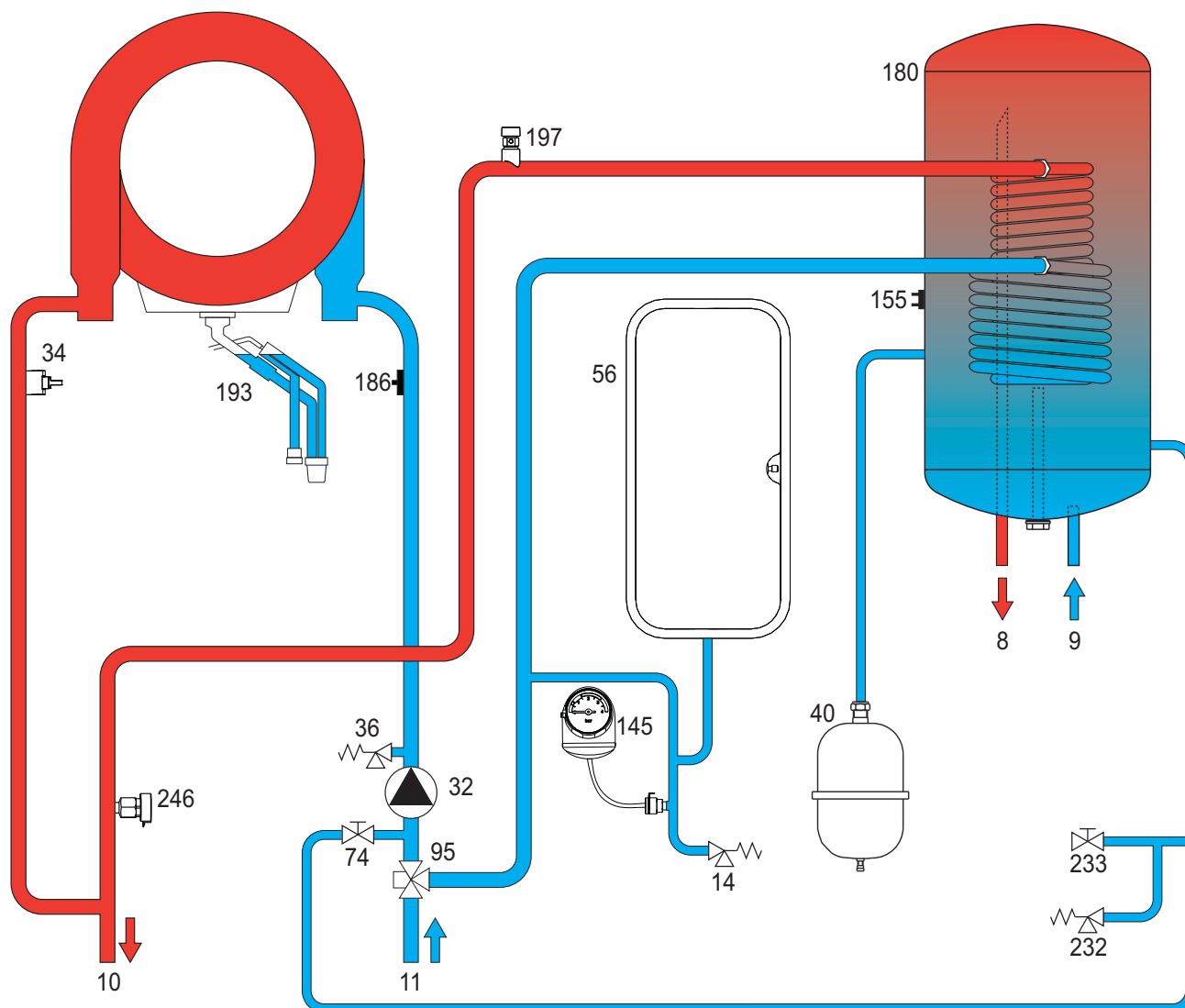
fig. 61 - Circuito idraulico
