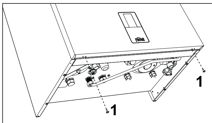
fig. 54 - Apertura pannello frontale
