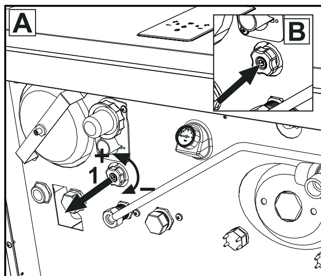
fig. 26- Filling knob
