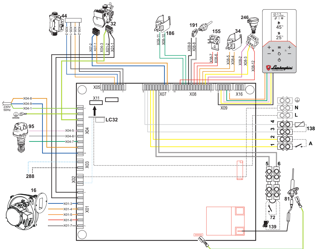
fig. 64- Wiring diagram
