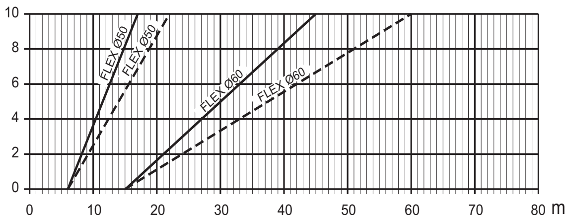
fig. 39- Gráfico para seleccionar el parámetro chimenea
