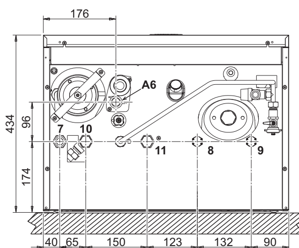
wygląd 59- Widok od dołu
