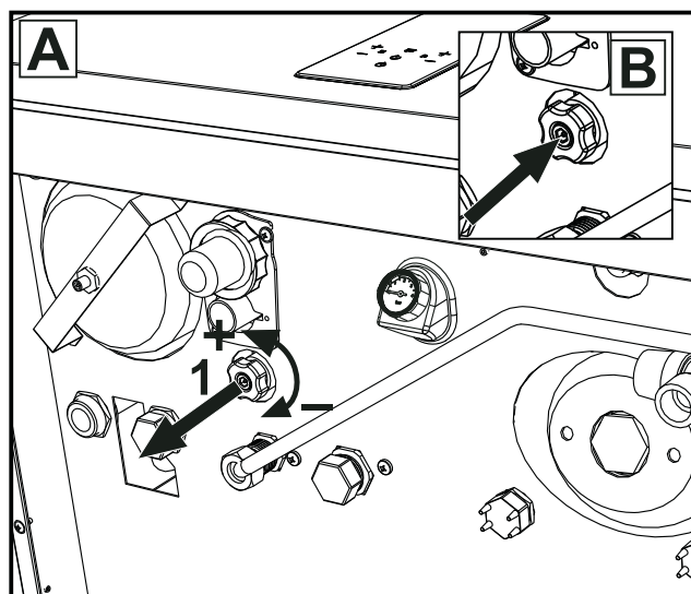
fig. 26 - Manopola di carico
