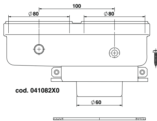
εικ. 35- Εξάρτημα σύνδεσης για ξεχωριστούς αγωγούς
