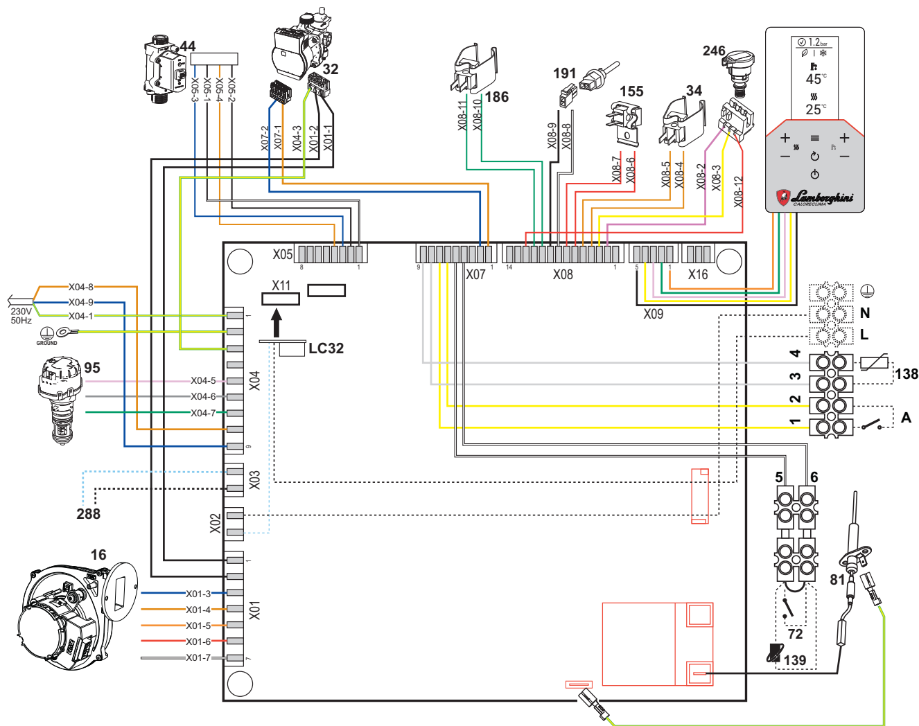
fig. 64- Schema electrică
