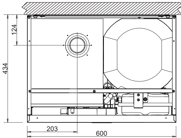
εικ. 58- Κάτωψη
