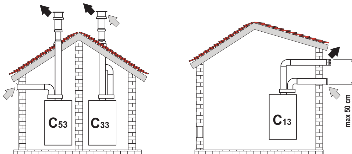
εικ. 34- Παραδείγματα σύνδεσης με ξεχωριστούς σωλήνες
